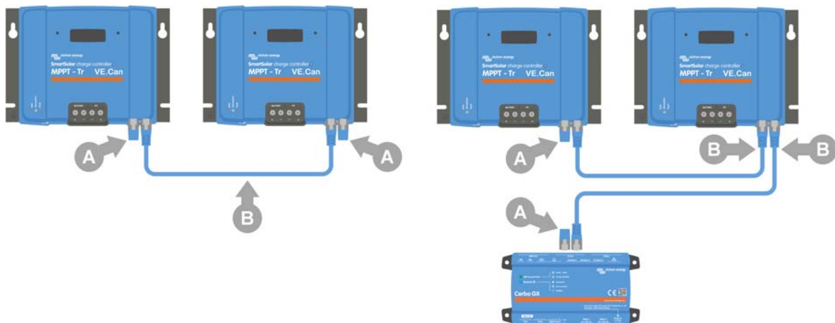
A: VE.Can terminator - B: RJ45 UTP cable.
